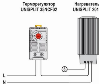
Рис. 2а - Пример подключения нагревателей UNISPLIT 201FXXX
