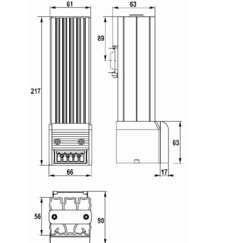
Рис. 1б – Общий вид и габаритные размеры нагревателей UNISPLIT 402SXXX
