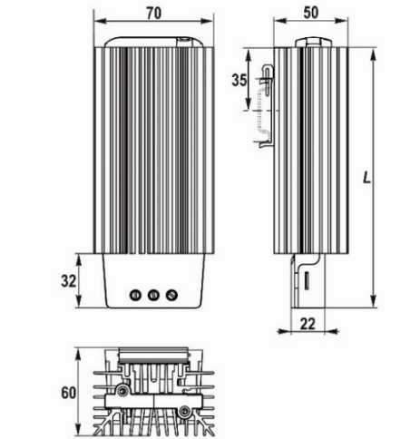
Рис. 1а – Общий вид и габаритные размеры нагревателей UNISPLIT 201FXXX
