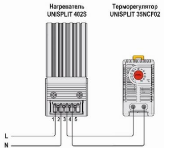
Рис. 2б - Пример подключения нагревателей UNISPLIT 402SXXX
