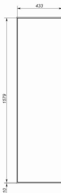
Монтажный вырез для наружного и полутопленного монтажа
