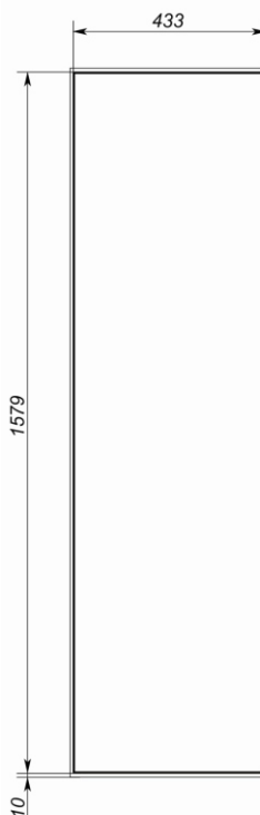
МОНТАЖНЫЙ ВЫРЕЗ наружный и полуутепленный монтаж
